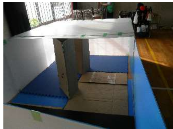
中に可動式の柱を置いたのがミソ（丈夫）。
